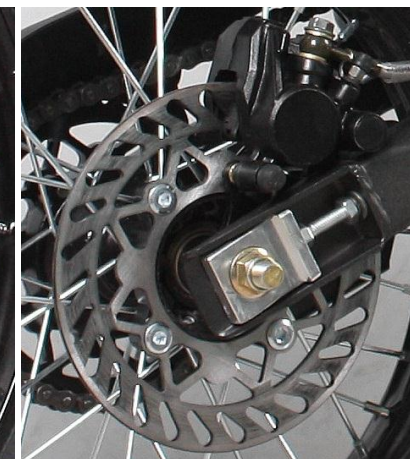
Задний тормоз
