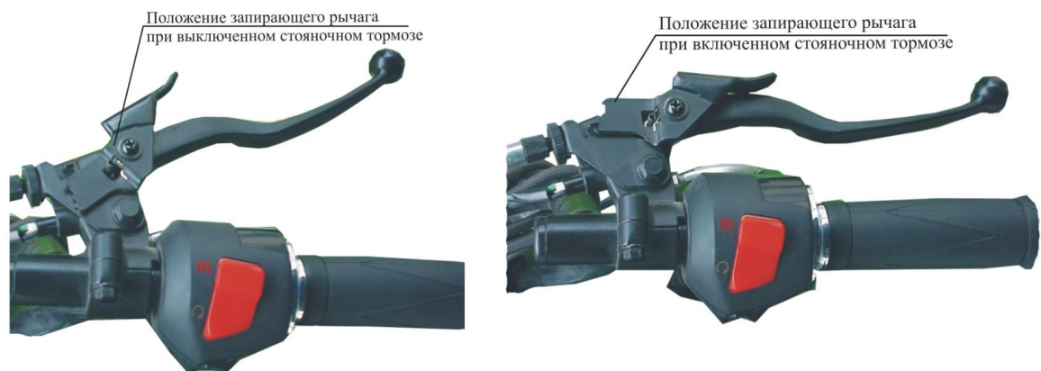
Рис. 13. Стояночный тормоз
