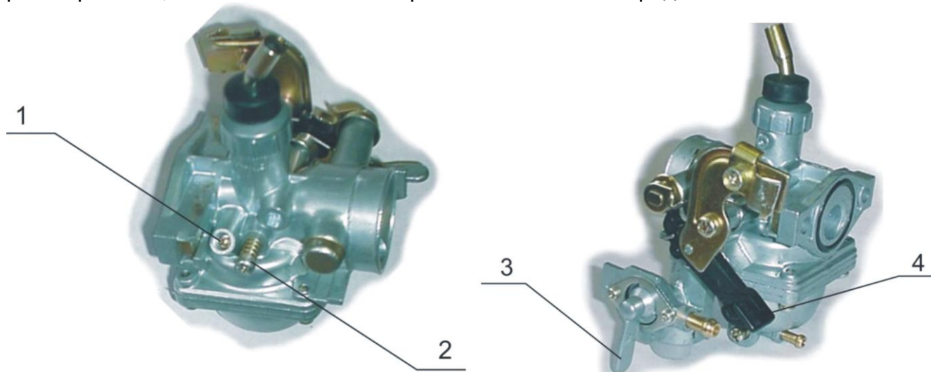
Рис. 5. Карбюратор
